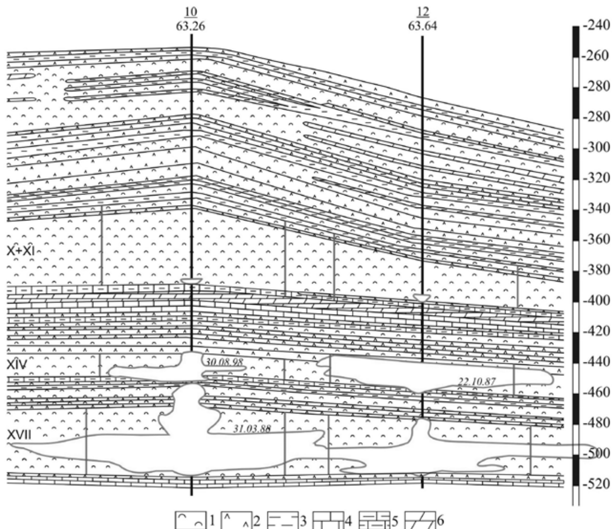
Рис. 2. Розріз через св. 10 та 12 Райгородської ділянки Слов'янського розсолотрому. Спотоворена форма камер та їх гідравлічний зв'язок (за матеріалами І. Н. Шевченко, 1952; С. В. Софроніної та ін.)
