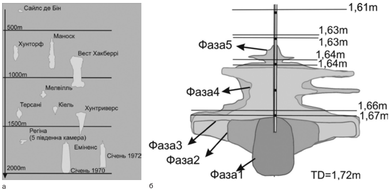
Рис. 1. Приклади форм камер, створених методом вилуговування у різних типах соленосних формацій (перерізи). Зіставлено об'єми ємності Емінінс, яка зазнала конвергенції (а). Зміна форми під час розмиву ємності Регіна (камера 5), що створена у девонській соленосній формації пластової форми залягання (Вінніпег, Канада) (б) [14, 15]
