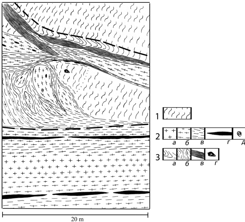
Рис. 2. Фрагмент контакту (очерчен пунктиром) структур етапу-1 с вязко-разломной структурой етапу-2 по короткій осі останньої. Зарисовка в плані.
