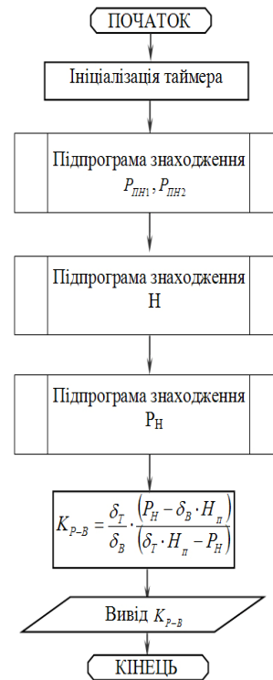
Рисунок 3 – Алгоритмічна схема знаходження K_{P/B}
