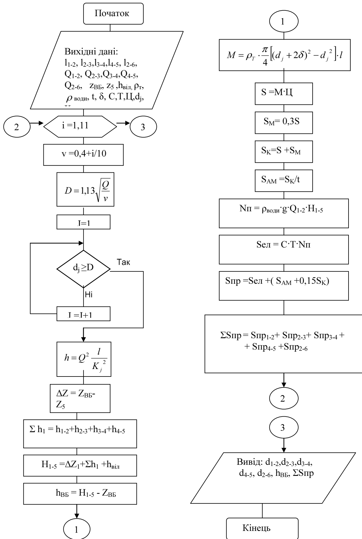
Рисунок 2 – Блок-схема алгоритму гідралічних і економічних розрахунків тупикової мережі водопостачання
