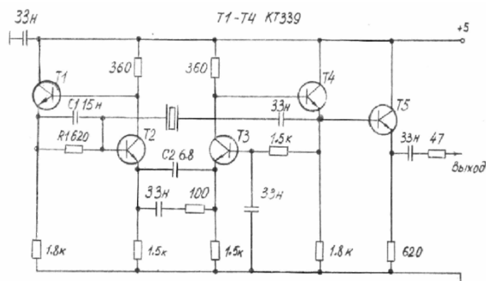
Рисунок 3 – Схема стабільного генератора
