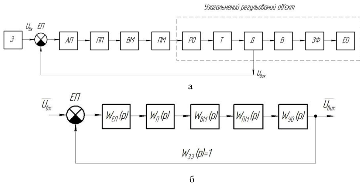
3 – задавач; АП – амплітудний підсилювач; ПП – підсилювач потужності; ВМ – виконавчий механізм; ПМ – перетворювальний механізм; РО – регулювальний орган; Т – трансформатор; Д – датчик; В – випрямляч; ЗФ – згладжувальний фільтр; ЕО – електромагнітна обмотка; W(p) – передавальні функції
