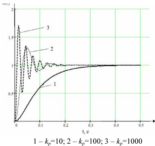
1 - k_p=10 ; 2 - k_p=100 ; 3 - k_p=1000 Рисунок 5 - Перехідні характеристики САК при різних значеннях коефіцієнта підсилення розімкнутої системи регулювання, що наближено дорівнює 0,4с. З підвищенням коефіцієнта підсилення розімкнутої системи до k_p = 100 перехідний процес стає коливальним і скорочується
