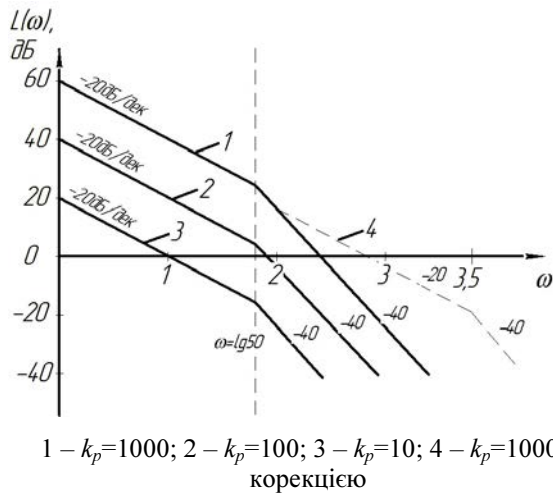
1 - k_p=1000 ; 2 - k_p=100 ; 3 - k_p=10 ; 4 - k_p=1000 з корекцією Рисунок 4 - Асимптотичні логарифмічні амплітудні частотні характеристики розімкнутої системи з різними коефіцієнтами підсилення
