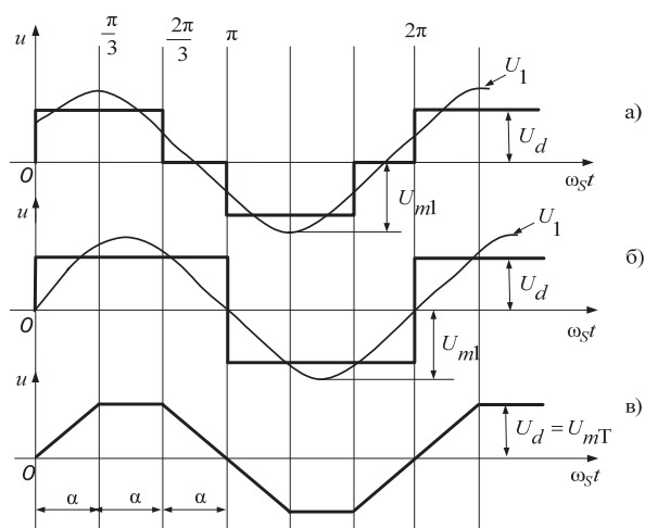
а) для трехфазного инвертора; б) однофазного моста при полном управлении; в) однофазного моста при трапецидальном управлении
