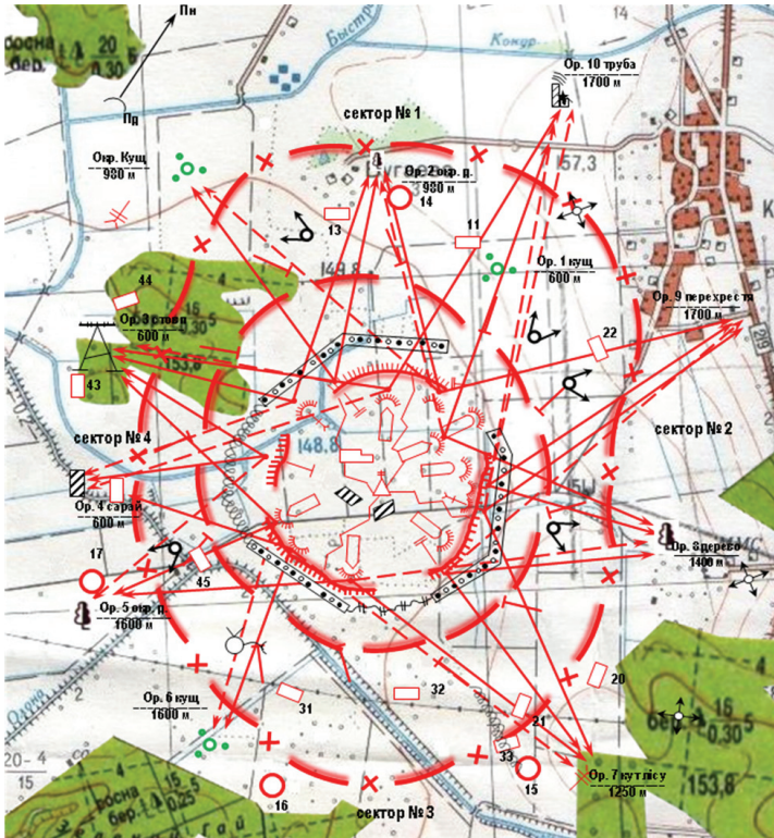
Варіант побудови оборони оперативно-бойової комендатури
