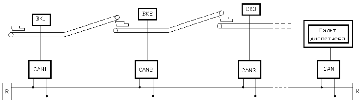
Рис. 1. Структурная схема сети передачи данных: ВК – видеокамера, CAN – контроллер, R – резисторы сопротивлением 120 Ом
