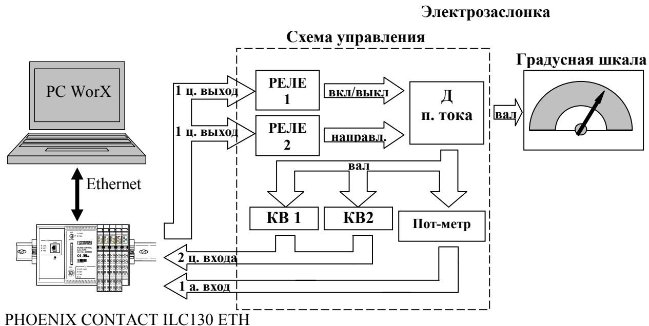
Рис. 4. Структура стенда управления электрзаслонкой
