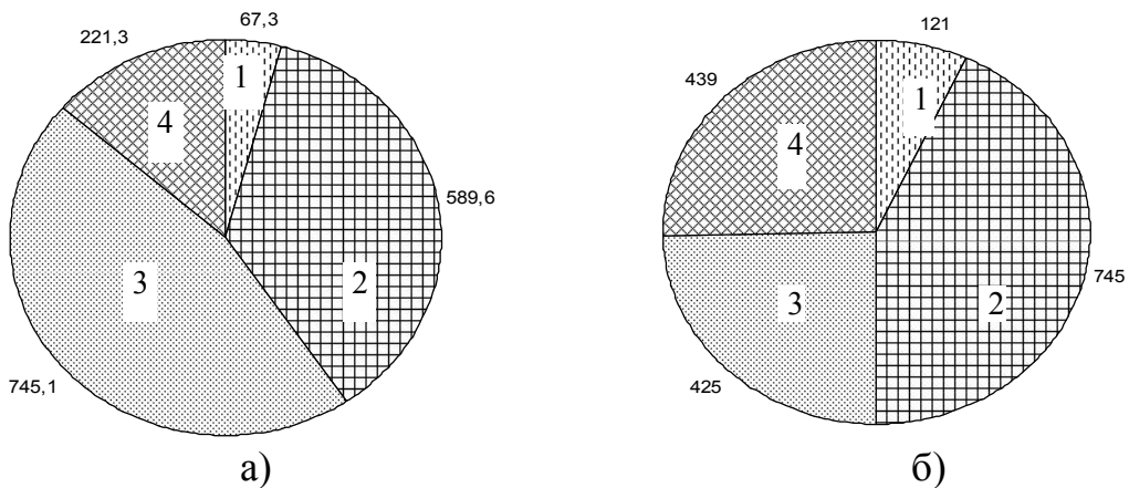
Рис. 5. Балансові складові підземних вод (м 3 /добу) до устаткування (а) і при роботі пропонованих дренажних заходів (б): 1 – надходження підземних вод за рахунок припливу з-за меж; 2 – надходження підземних вод за рахунок інфільтрації; 3 – витрати підземних вод на межах; 4 – перетікання підземних вод у другий водоносний горизонт
