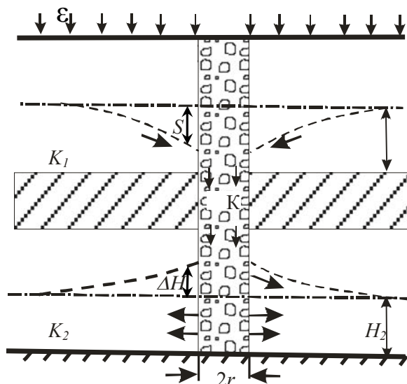
Рис. 1. Схема вертикальної поглинаючої свердловини: S – пониження рівня ґрунтових вод; H_1 , H_2 , K_1 , K_2 – відповідно потужність верхнього і нижнього водоносного горизонту та їх коефіцієнти фільтрації; r_0 – радіус ствола свердловини заповненого матеріалом з коефіцієнтом фільтрації K ; \Delta H_2 – підвищення рівня підземних вод в нижньому горизонті; \epsilon – інфільтраційне живлення
