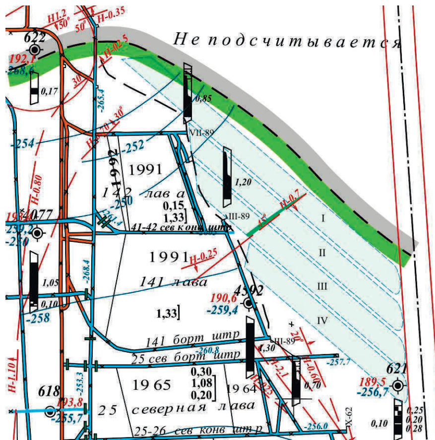
Рис. 2. План ділянки № 2 для впровадження технології СПГВ
