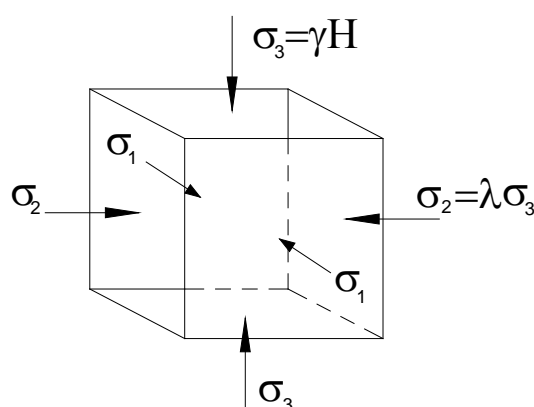
Рис. 2. Схема напряженного состояния элементарного объема массива горных пород при отсутствии влияния очистной выработки
