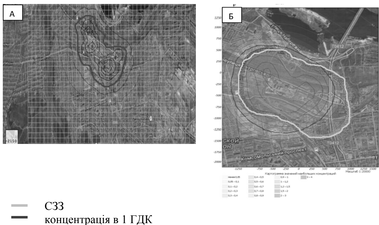
Рис. 3. Карта розсіювання цементного пилу А) оригінальне зображення за «ЕОЛ+» накладене на космоснімок місцевості; Б) карта розсіювання цементного пилу (УПРЗА «Еколог»)
