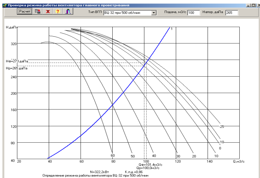
Рис. 3. Графическая интерпретация результатов расчета: 1 - аэродинамическая характеристика ШВС
