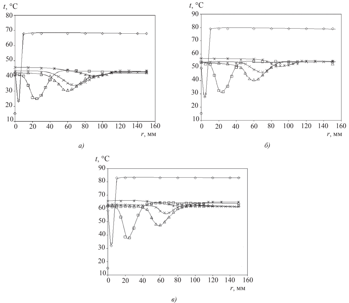
Рис. 3. Розподіл температур по перерізу каналу для P = 0,6 \text{ МПа} , V = 19,5 \text{ м}^3/\text{год} при різних об'ємних долях пари в суміші \varepsilon (а — \varepsilon = 0,1 ; б — \varepsilon = 0,2 ; в — \varepsilon = 0,3 ) на різних висотах від зрізу сопла форсунки і величинах h = 11 \text{ мм} ; 2 — 40 мм; 3 — 90 мм; 4 — 110 мм; 5 — 190 мм; б — температура води перед соплом форсунки ( h = 0 ):
