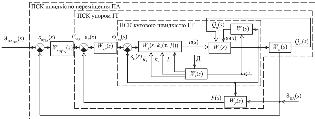
Рис. 2. Структурна схема САК швидкістю переміщення ПА за його горизонтального прямолінійного руху:
