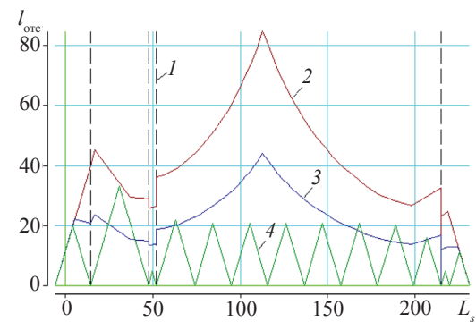
Рис. 2. Кривая предельных длин отсеков
