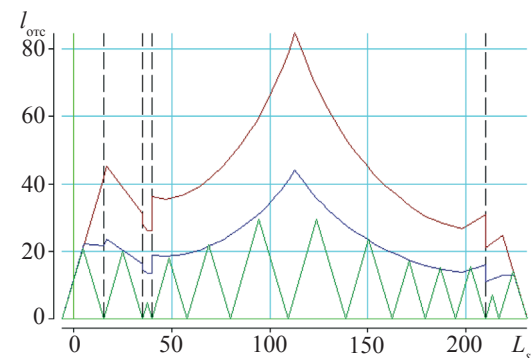
Рис. 3. Кривая предельных длин отсеков после смещения переборок
