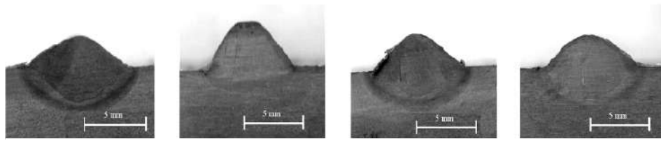
Рис. 3. Макрошлифы валков, наплавленных с разными параметрами режима ИПЭП
