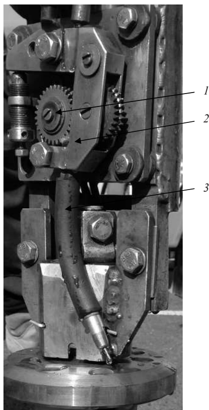
Рис. 7. Сварочная горелка с колебателем: 1 — эксцентрично установленный подающий ролик; 2 — прижимной рычаг; 3 — колебатель
