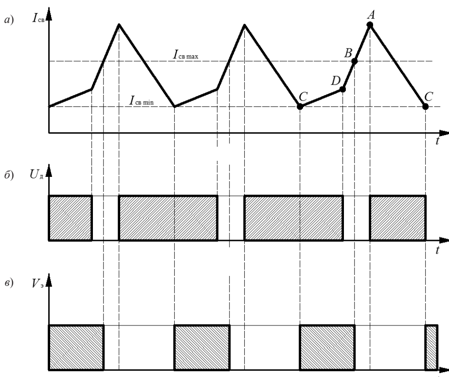
Рис. 5. Алгоритм работы системы управления переносом электродного металла, связанной с параметрами дугового процесса: a — схематизированная осциллограмма сварочного тока I_{св} ; б — схематизированная осциллограмма напряжения на дуге U_d ; в — циклограмма работы электропривода ( v_w — скорость подачи электродной проволоки); A — начало перехода капли электродного металла в сварочную ванну; B и C — моменты достижения сварочным током установленной максимальной и минимальной величины соответственно; D — начало короткого замыкания дугового промежутка
