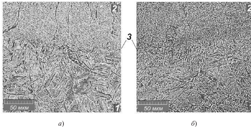
Рис. 4. Микроструктура стали (данные электронной микроскопии, \times 1000 ) в районе линии сплавления при подаче электродной проволоки: a — с постоянной скоростью; б — в импульсном режиме; 1 — основной металл (09Г2С); 2 — наплавленный металл (30ХГСА); 3 — линия сплавления
