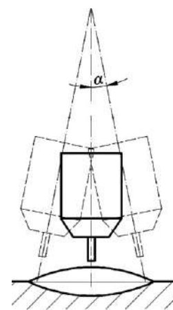
Рис. 8. Схема внеосевых колебаний электродной проволоки
