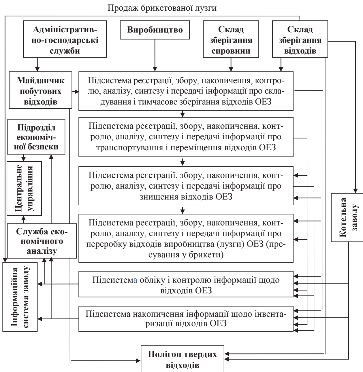
Рис. 2. Узагальнена схема структури інформаційної системи управління відходами ОЕЗ (Джерело: власна розробка автора)
