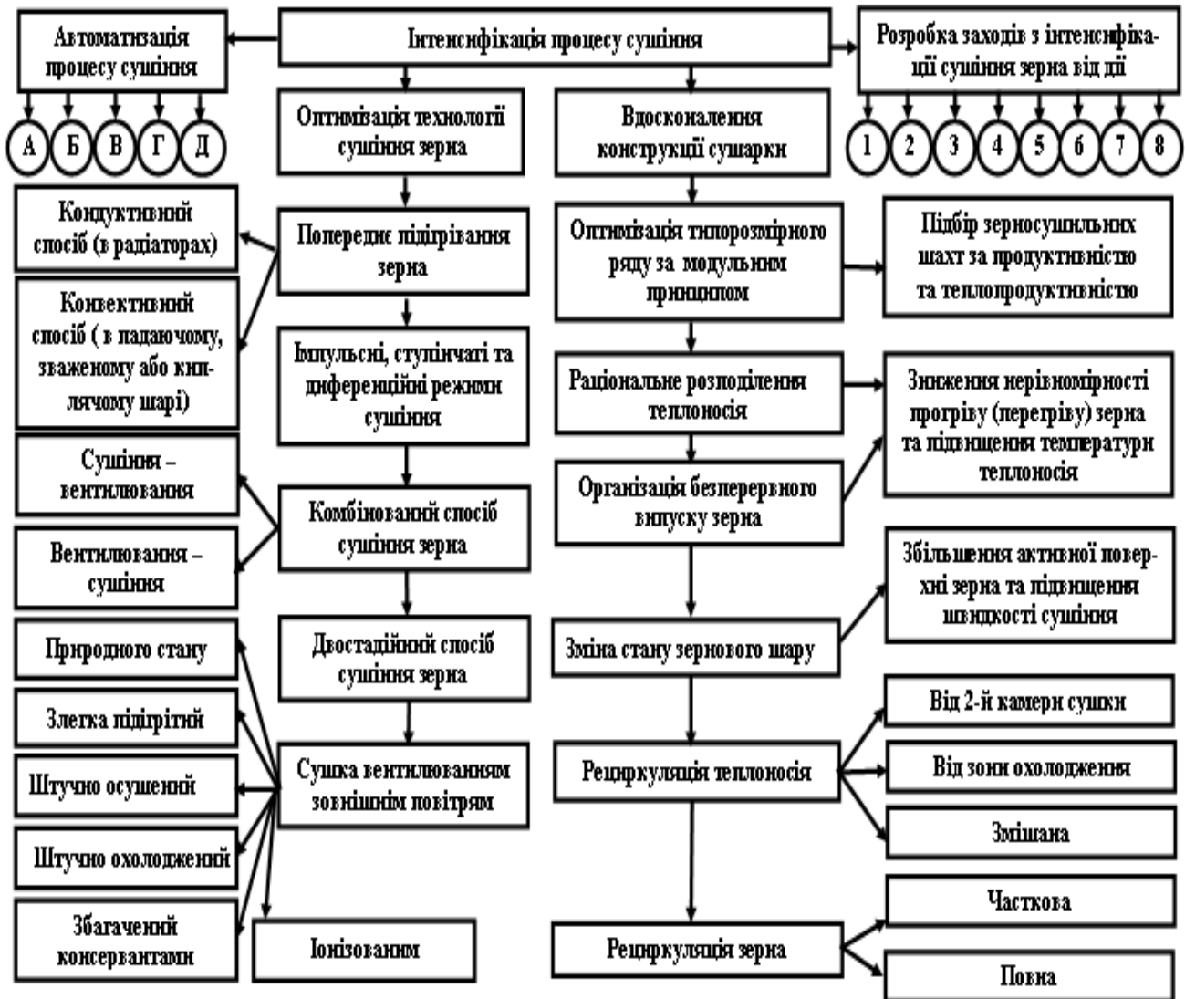
Рис. 2. Класифікація основних шляхів інтенсифікації сушіння зерна. контроль та вимірювання:
