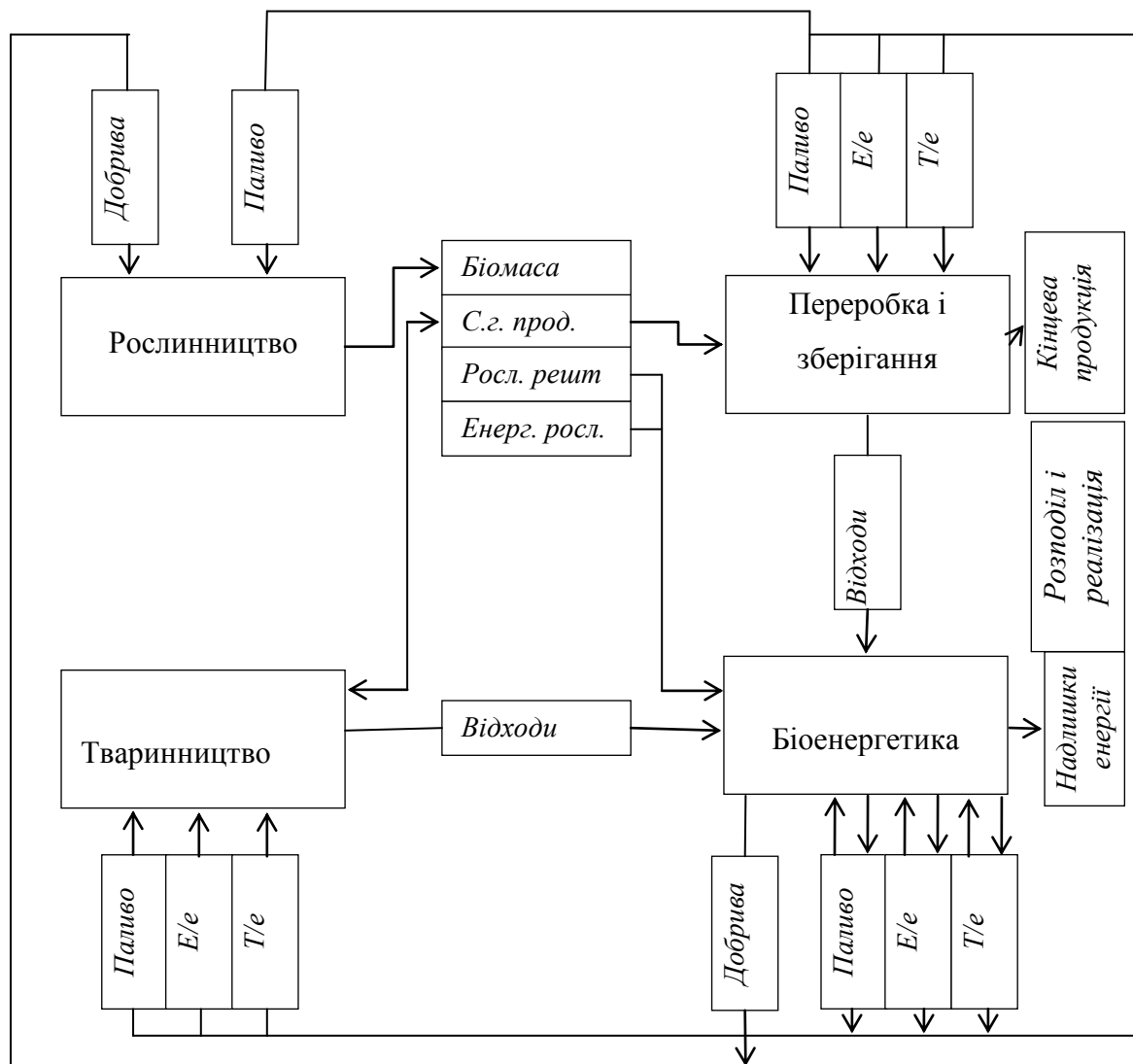
Рис. 2 Схема кругообігу енергії та речовин комплексної агробіоінженерної системи виробництва та використання біопалива, де: e/e – електроенергія, t/e – теплова енергія
