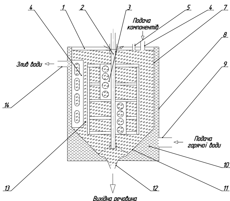
Рис. 2 - Схема змішувача для одержання «грубої» емульсії маргарину
