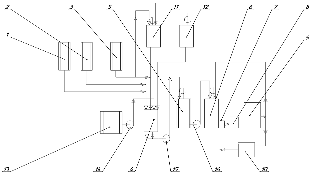
Рис. 1 - Апаратурно-технологічна схема виробництва маргарину
