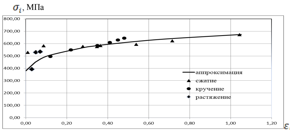
Рис. 3. Кривая течения стали 20
