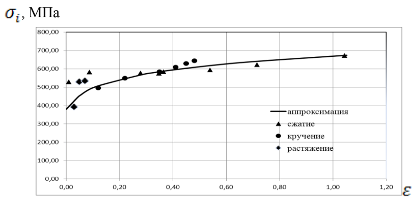
Рис. 3 Кривая течения стали 20
