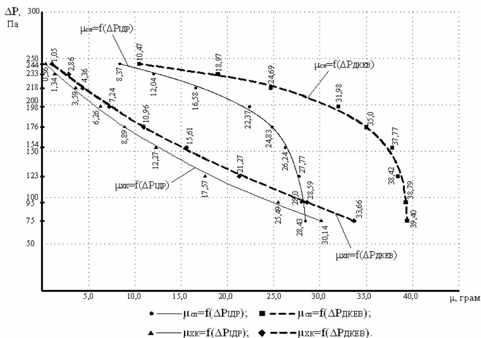
Рис. 6. Графіки залежності кількості вловлених транспортуючих компонентів сояшнікової лузги \mu_{СЛ} та хлібної крихти \mu_{ХК} від втрат тиску \Delta P на регулюючих пристроях різних конструктивних виконань
