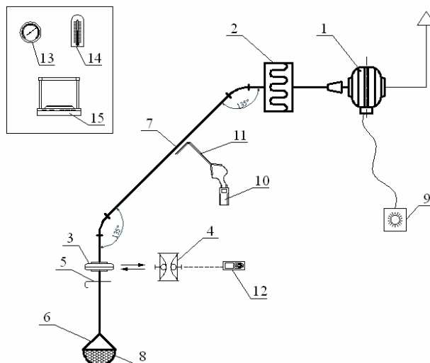
Рис. 1. Конструктивна схема експериментальної установки
