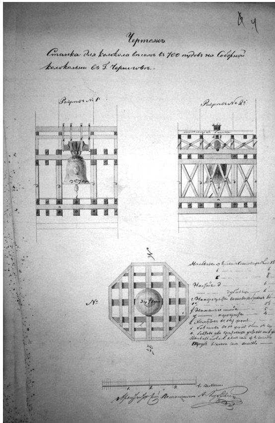
Рис. 1. Кресленник нового станка для дзвону «Борис» (Державний архів Чернігівської області, ф. 179, оп. 30, спр. 140, арк. 4. Оригінал)
