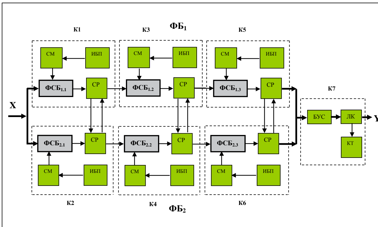
Рис. 2. Инфраструктурная схема СПА повышенной живучести на СДКМС
