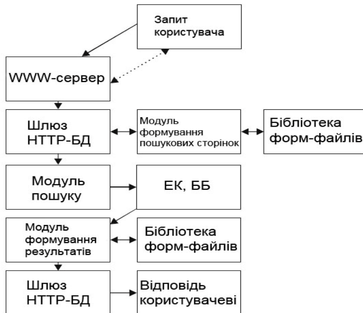
Рис. 2. Загальна функціональна блок-схема алгоритму роботи Web-IPBIS 64 [8]
